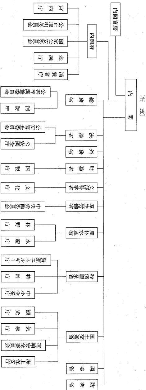
行政機構圖
